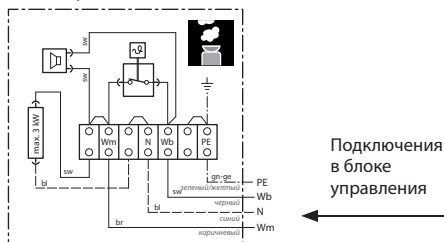
Испаритель
